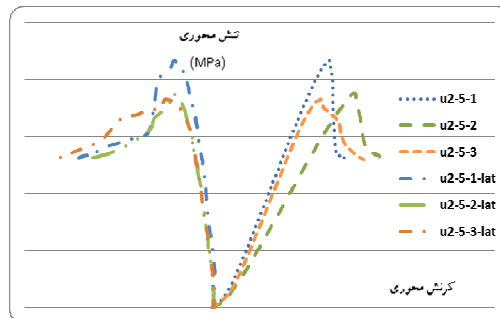
شکل ۱۴- منحنی‌های تنش-کرنش محوری و جانبی برای بتن فوق-توانمند حاوی دو درصد الیاف (U۲) در فشار جانبی ۵ مگاپاسکال
