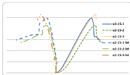
شکل ۱۶- منحنی‌های تنش-کرنش محوری و جانبی برای بتن فوق-توانمند حاوی دو درصد الیاف (U۲) در فشار جانبی ۱۵ مگاپاسکال
