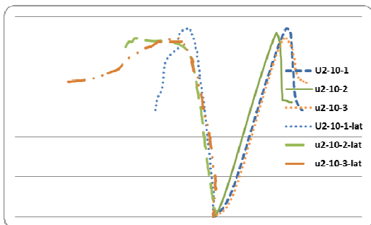
شکل ۱۵- منحنی‌های تنش-کرنش محوری و جانبی برای بتن فوق-توانمند حاوی دو درصد الیاف (U۲) در فشار جانبی ۱۰ مگاپاسکال
