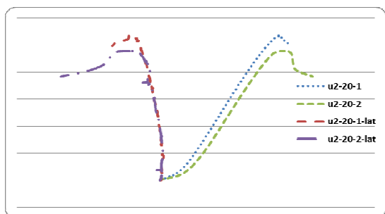
شکل ۱۷- منحنی‌های تنش-کرنش محوری و جانبی برای بتن فوق-توانمند حاوی دو درصد الیاف (U۲) در فشار جانبی ۲۰ مگاپاسکال
