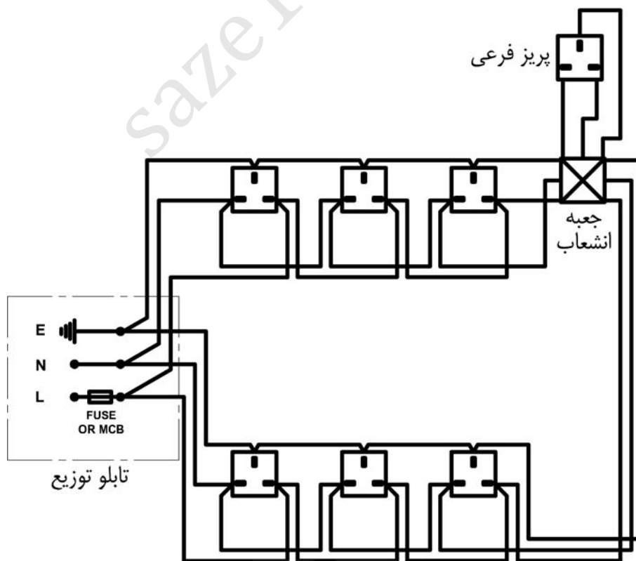
شکل ۲-۳: سیستم سیم‌کشی حلقوی مدار پریزها
