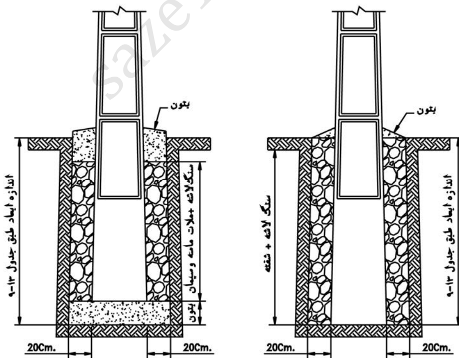
۱۳-۱۰: نصب پایه‌های انتهایی، زوایا، و نگهدارنده ترانسفورماتور
