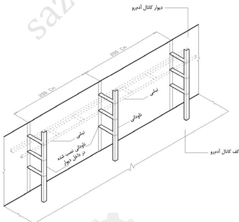
شکل ۸-۳: جزئیات تیپ اسکله‌بندی نصب کابل در داخل کانال‌های آدرو
