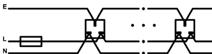
شکل ۱-۳: سیستم سیم‌کشی شعاعی مدار پریزها
