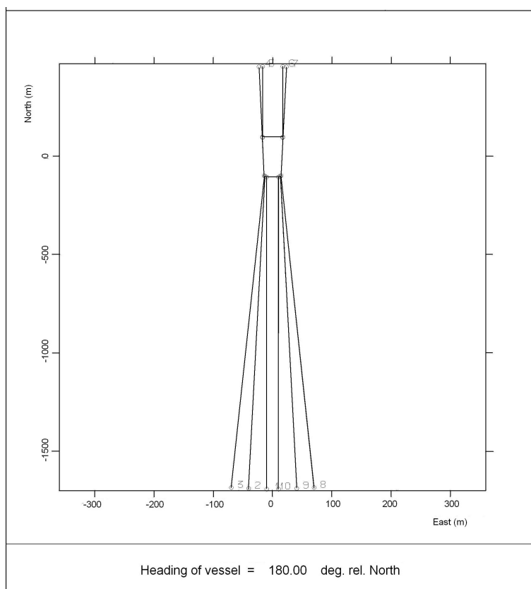
شکل ۴- نمای الگوی مهاربندی بهینه شده برای شرایط محیطی تک جهته به سمت شمال
