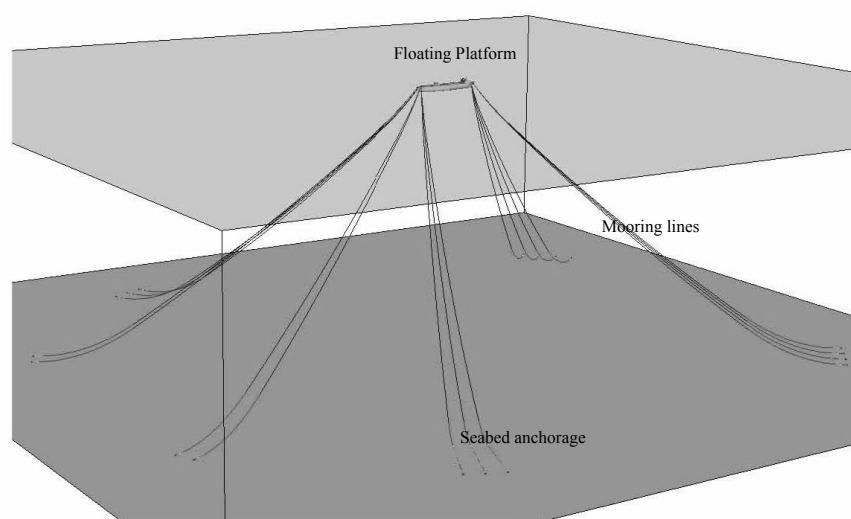
شکل ۱- نمایی از سیستم مهاربندی کتتری
