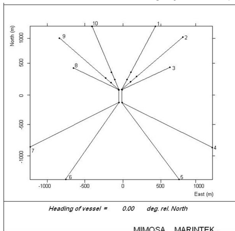
شکل ۳- نمای الگوی مهاربندی کتتری حول یک سکوی FPSO شامل ۱۰ خط مهار
