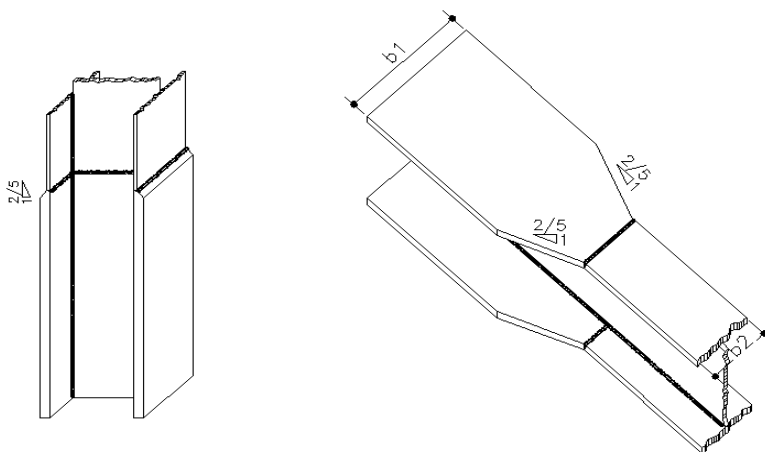
تغییر تدریجی ابعاد مقطع در وصله، با شیب 2/5 : 1
