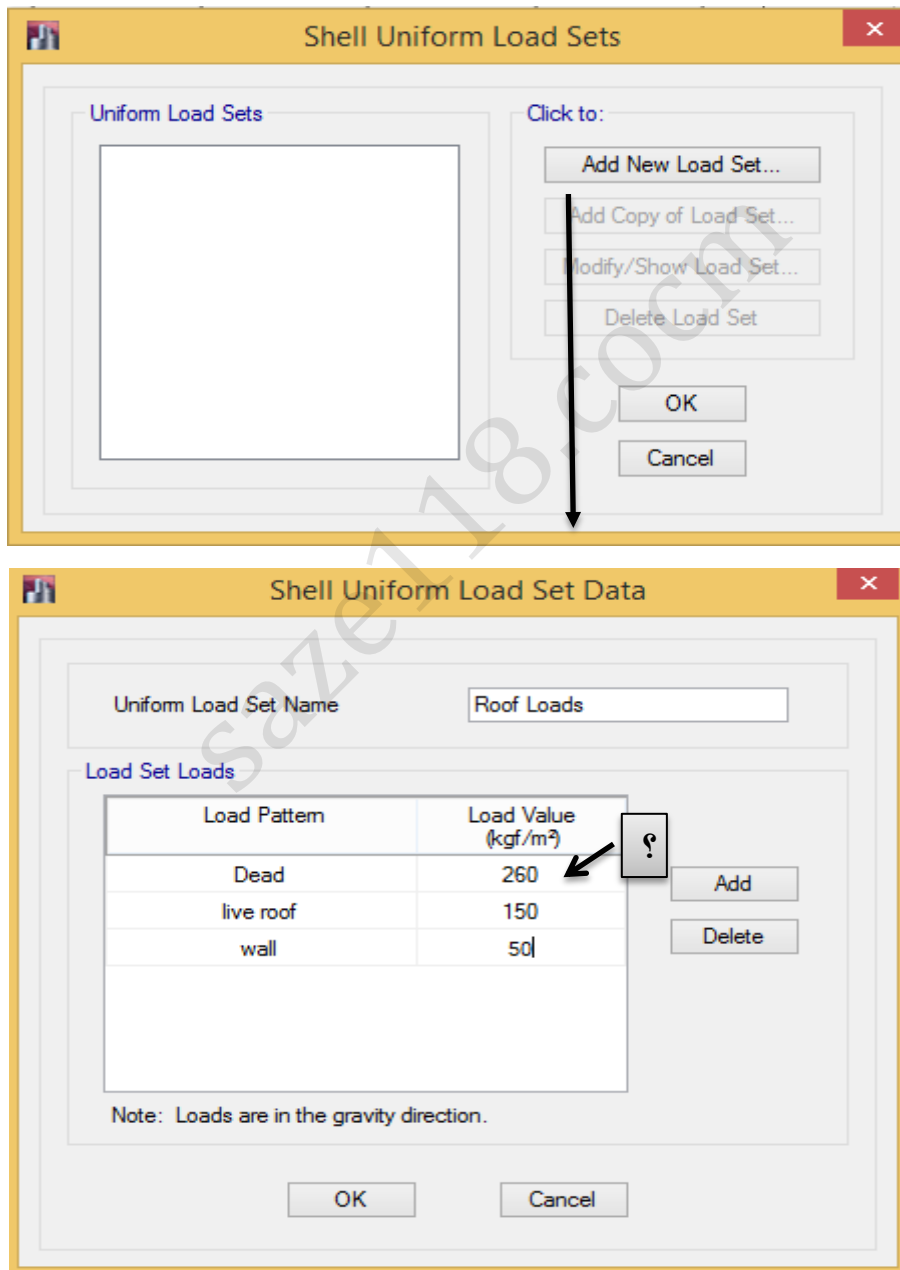
شکل ۷۳: بسته بارگذاری گسترده بام
