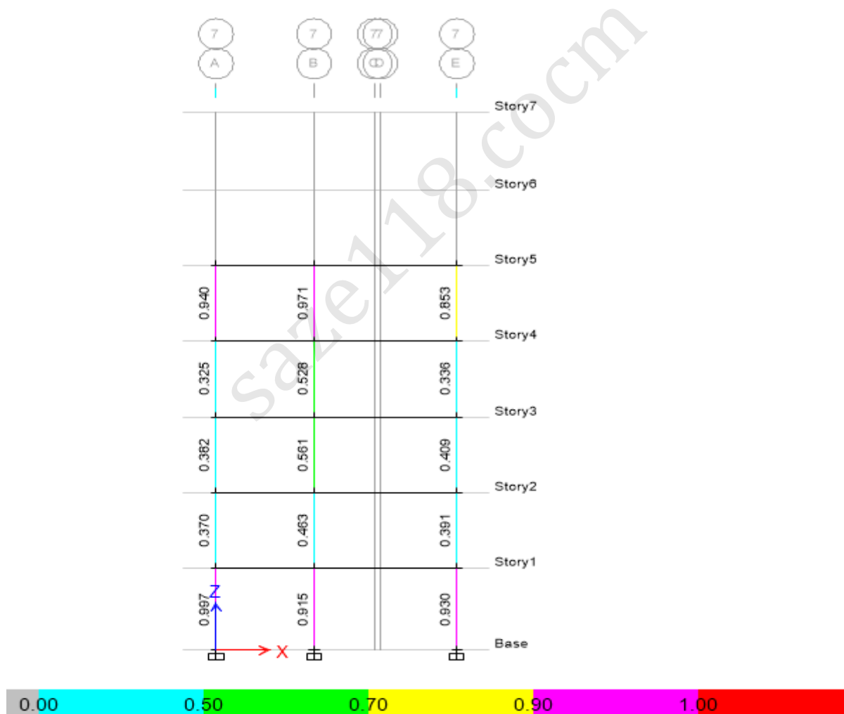
شکل ۹۴: نمایش Ratios و کفایت ستونها
