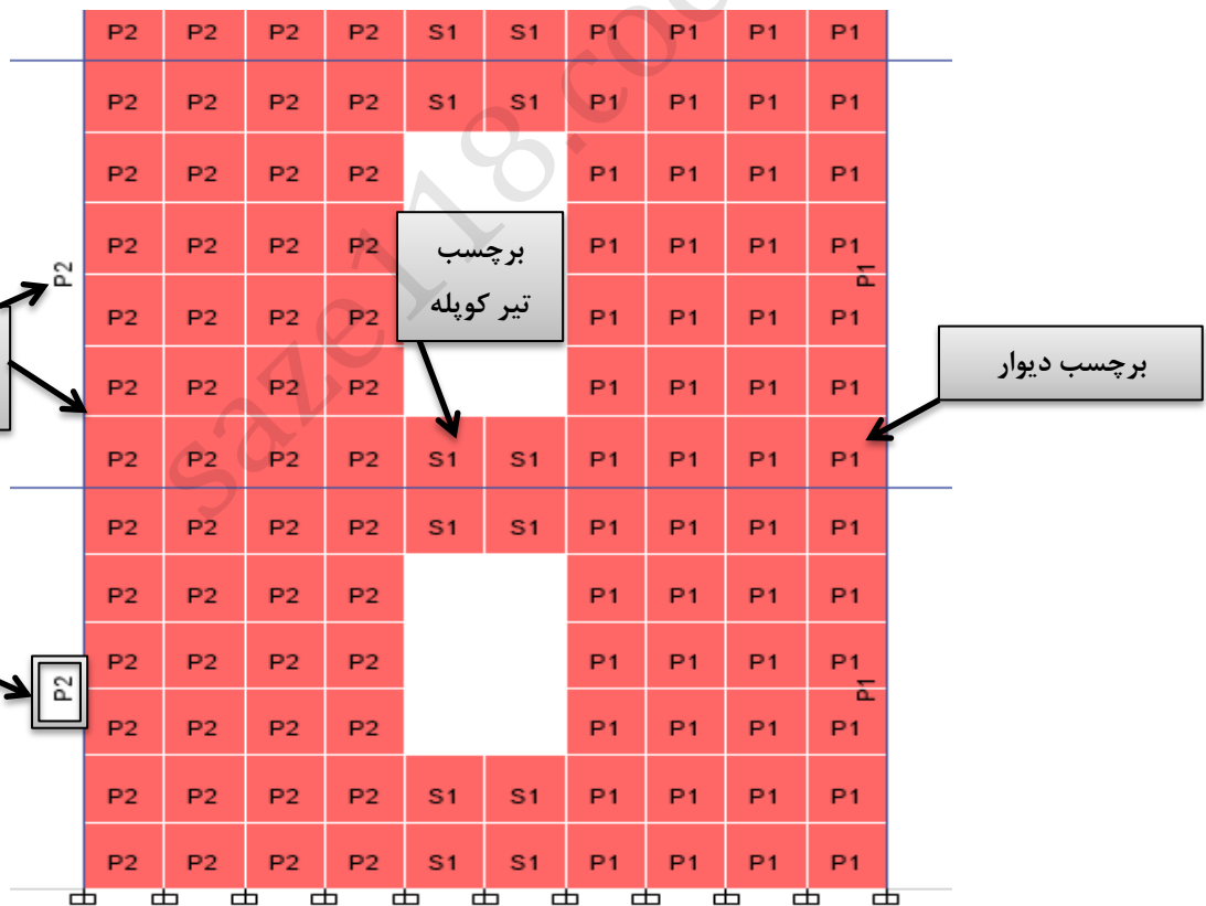
شکل ۱۰۳: نامگذاری دیوارها و تیر پیوند
