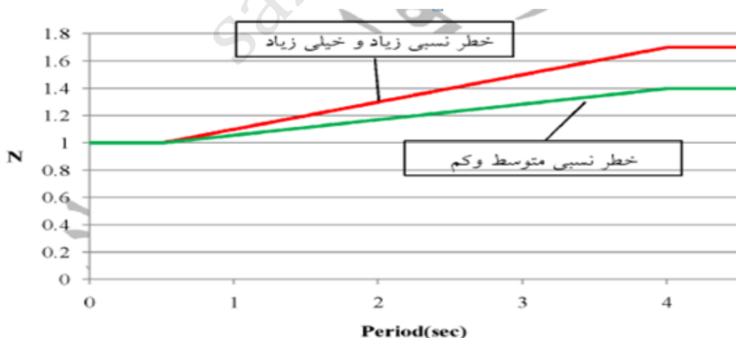
شکل ۲۳: ضریب اصلاح طیف، N برای پهنه‌های با خطر نسبی خیلی زیاد، زیاد، متوسط و کم
