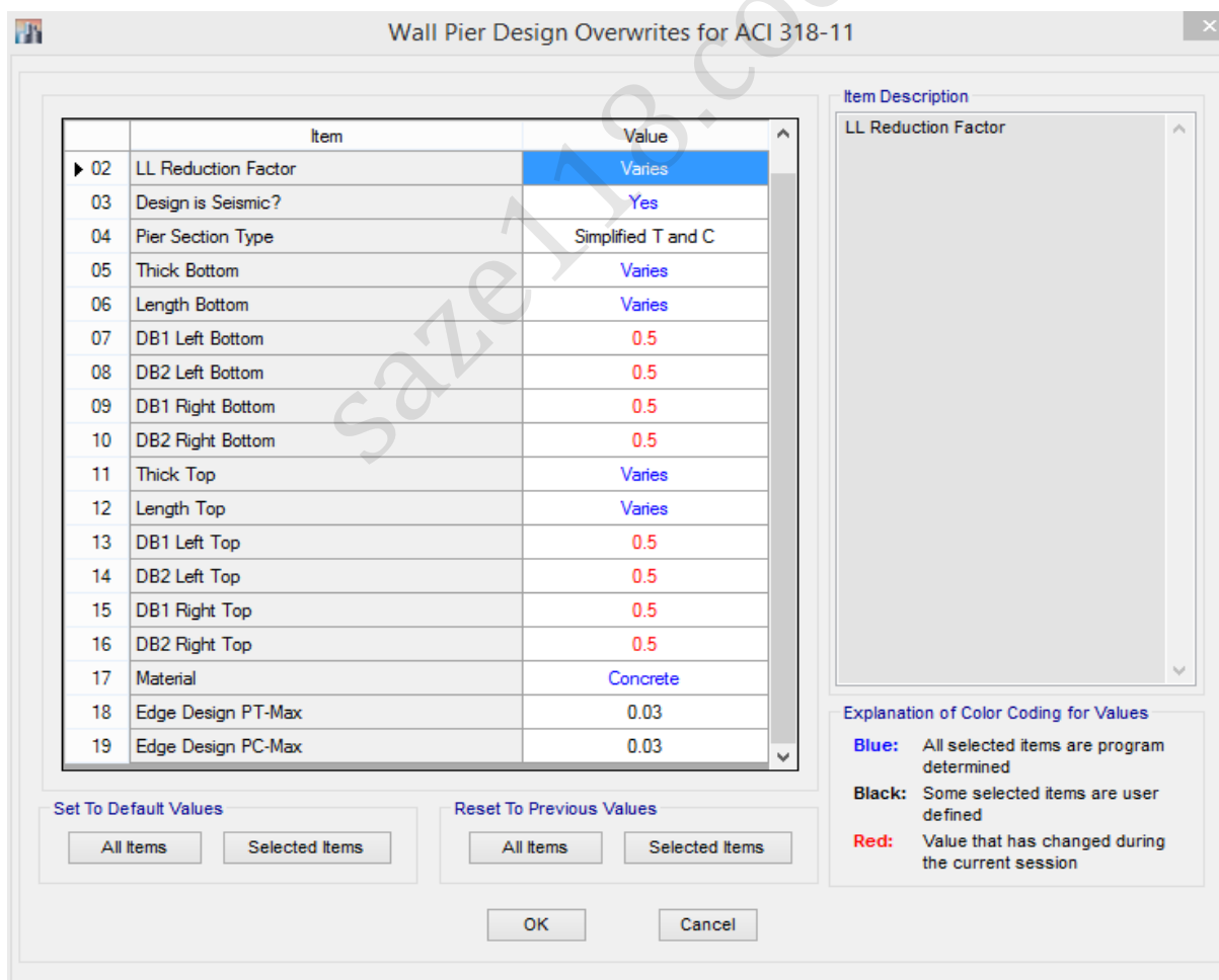
شکل ۱۰۵: تنظیمات مربوط به طراحی دیوار
