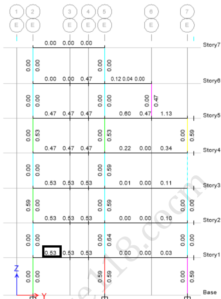
شکل ۹۶: نمایش \frac{A_v}{s} میلگردهای عرضی
