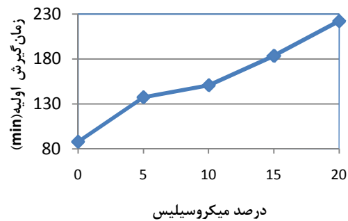
شکل ۱۴- نمودار زمان گیرش اولیه (بر حسب دقیقه) برای نمونه‌های حاوی درصد‌های مختلف میکروسیلیس
