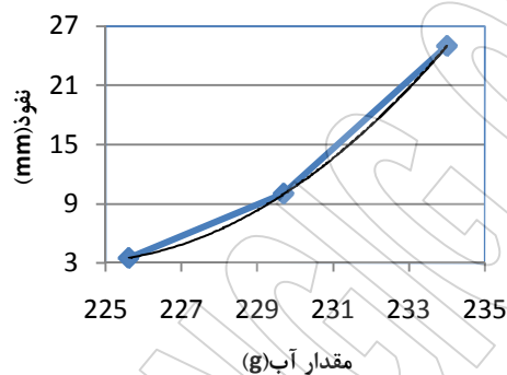
شکل ۵- نمودار آزمایش غلظت نرمال برای سیمان ۸۰٪
