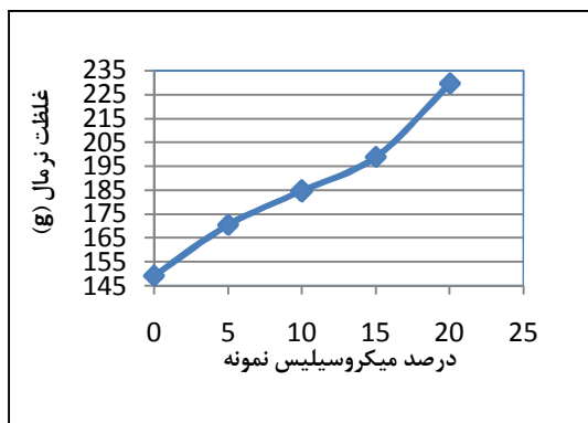
شکل ۶- نتایج آزمایش غلظت نرمال؛ غلظت نرمال آب در برابر درصد میکروسیلیس نمونه
