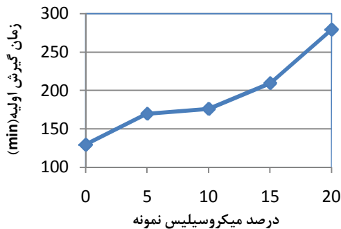
شکل ۲۰- زمان گیرش نهایی بر حسب درصد میکروسیلیس
