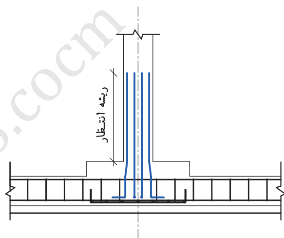
◀ مرحله شماره (۲)
