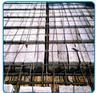
شکل ۷-۳۴- میلگردهای افت و حرارت
