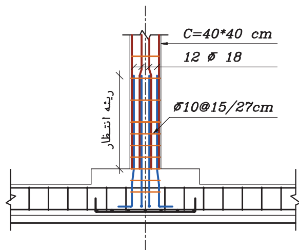
◀ مرحله شماره (۴)
