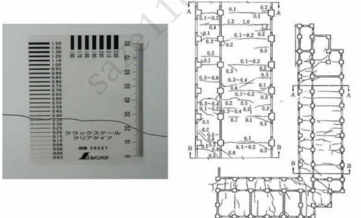
ب- پلان سازه
