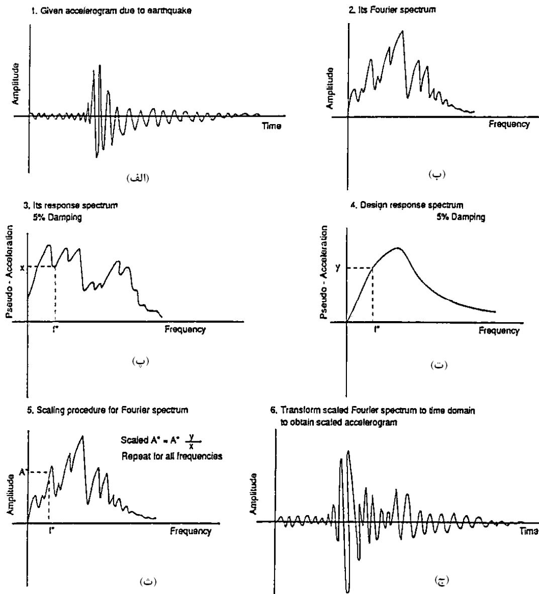
شکل ۳-۵- مراحل مختلف تهیه تاریخچه زلزله براسای طیف پاسخ طرح
