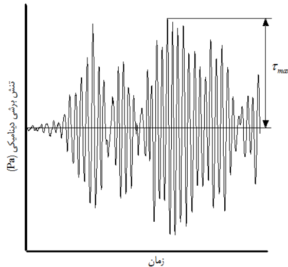
شکل ۳-۵۲- تاریخچه تنش برشی تناوبی و حداکثر تنش برشی در تحلیل دینامیکی
