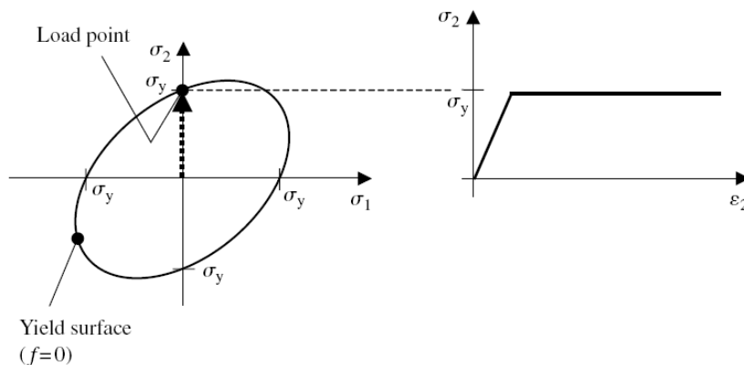
شکل ۳-۱۶- یک نوع سطح تسلیم در مدل‌های الاستوپلاستیک کامل و رفتار تنش - کرنش مربوطه
