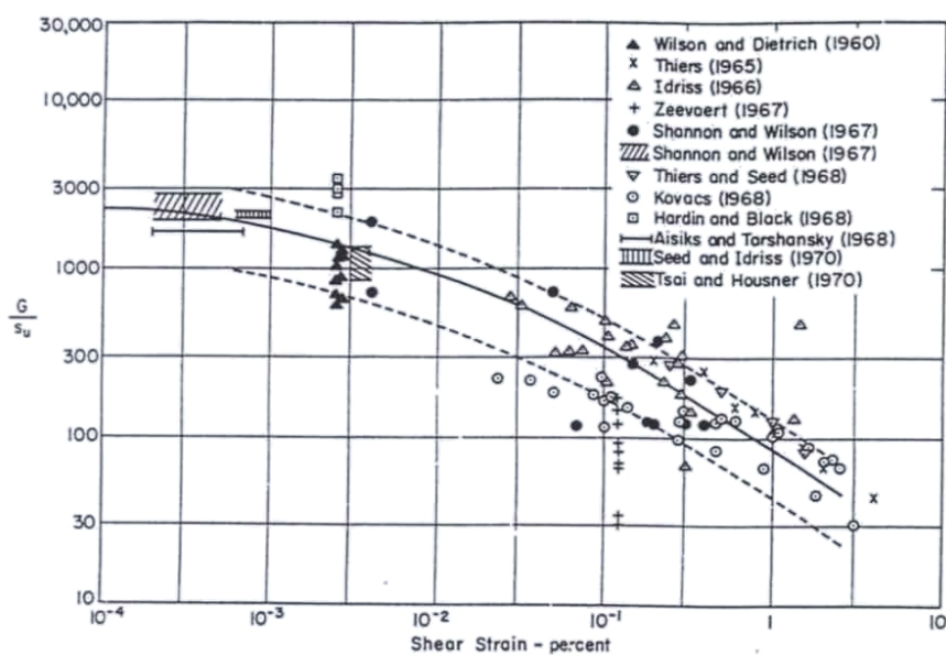
شکل ۲۶-۳- تغییرات مدول برشی با کرنش برشی در خاک رسی اشباع
