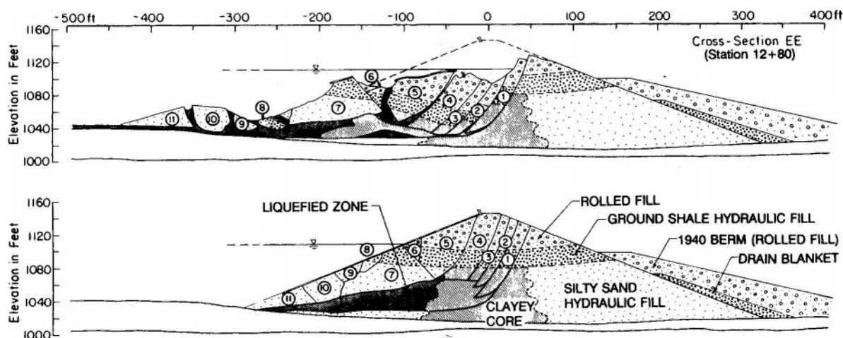
شکل پ-۱-۱- مقطع عرضی سد سن فرناندوی پایینی در زلزله ۱۹۷۱ و مقطع عرضی اولیه
