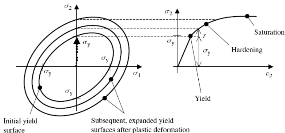
شکل ۳-۱۹- یک نوع سطح تسلیم در مدل‌های الاستوپلاستیک سخت شونده و رفتار تنش - کرنش مربوطه
