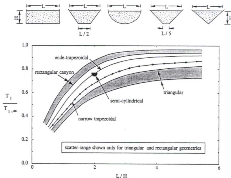
شکل ۳-۱۰- اثر هندسه دره در پرورد طبیعی سد خاکی
