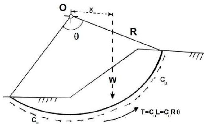
شکل ۶-۲- نیروهای وارد بر یک سطح لغزش دایره‌ای در روش سوئدی ( \theta = 0 )
