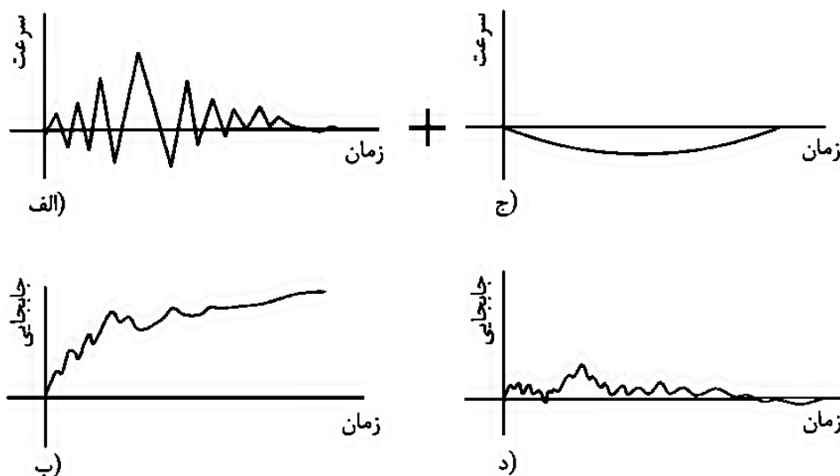
شکل ۳-۸- نحوه اصلاح خط مبنا
