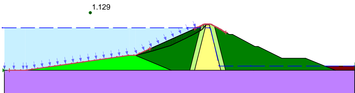
شکل پ ۸-۴۴ - سطح لغزش بحرانی شیب بالادست در تحلیل شبه استاتیکی مرحله تراوش پایدار از مخزن نیمه پر تحت زلزله MDE - مقطع میانی سد (تراز نرمال آب مخزن - ۱۷۱ متر)
