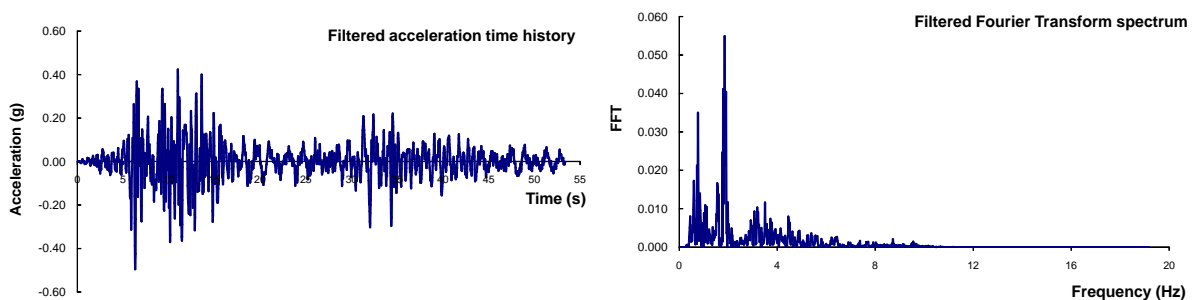
شکل پ ۸-۶۰- تاریخچه زلزله فیلتر شده و طیف دامنه فوریه آن با محو شدن فرکانسهای بالای ۱۰ هرتز
