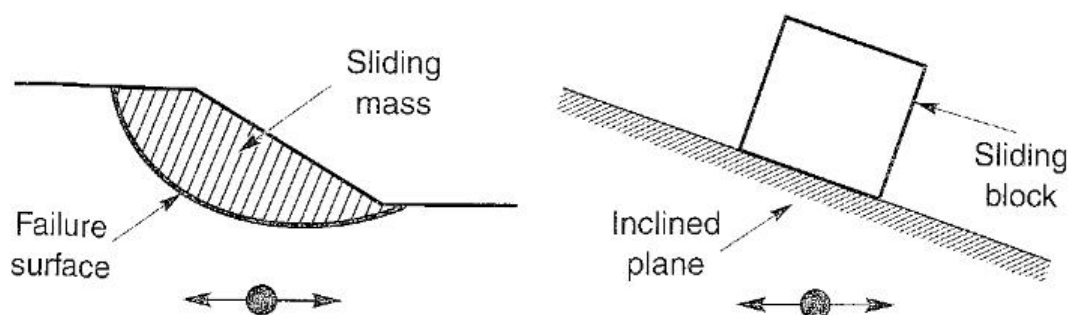
شکل ۳-۳۸- همانندی بین توده لغزشی و بلوک لغزش نیومارک بر روی سطح شیب‌دار
