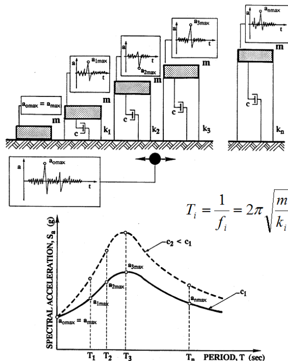
شکل ۲-۳-۲- مفهوم طیف پاسخ
