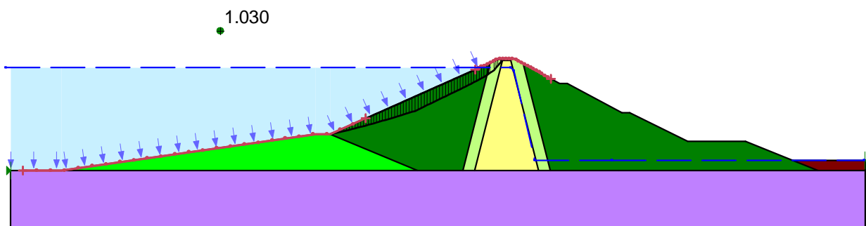
شکل پ ۸-۴۵ - سطح لغزش بحرانی شیب بالادست در تحلیل شبه استاتیکی مرحله تراوش پایدار از مخزن نیمه پر تحت زلزله MCE - مقطع میانی سد (تراز نرمال آب مخزن - ۱۷۱ متر)
