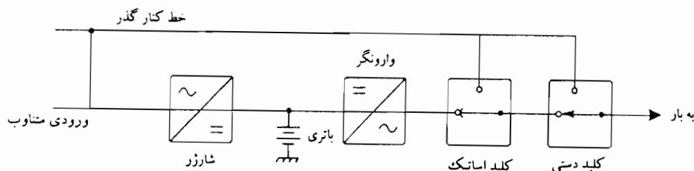
شکل ۸-۴ الف - سیستم یو - پی - اس از نوع ایستا با کلیدهای کنار گذر
