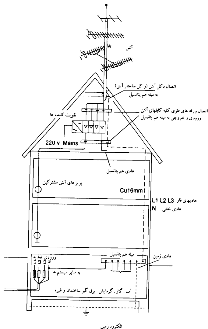
شکل ۴-۱۳ هم پتانسیل نمودن آنتن همگانی با سایر اجزای فلزی ساختمان
