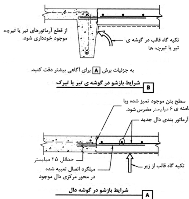
شکل ۱۰-۱- پر کردن بازشو در دیافراگم بتنی
